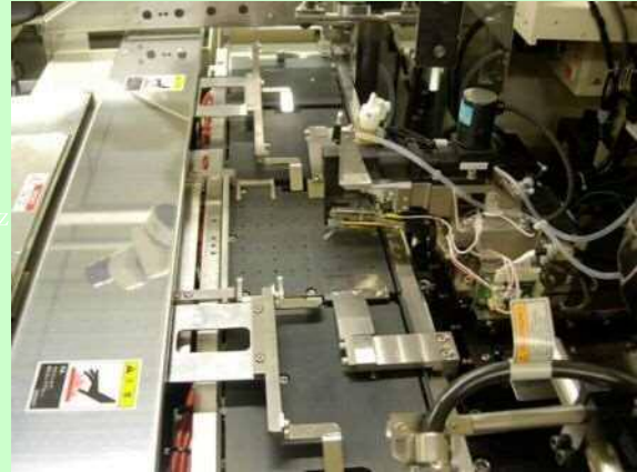
個片基板(キャリア搬送)
